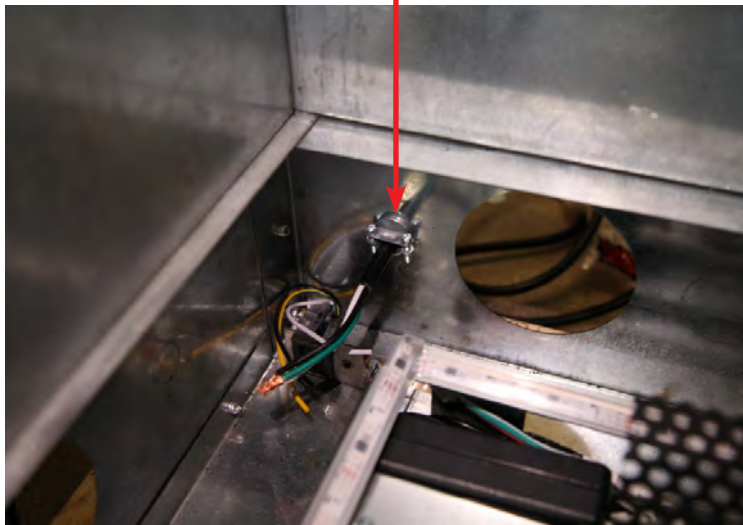
Conduit clamp
