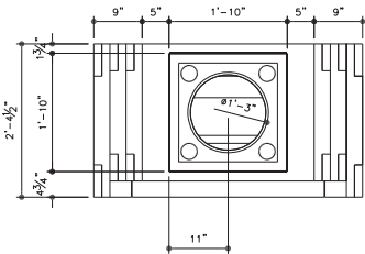
CHIMNEY PLAN SCALE: 1" = 1'-0"
